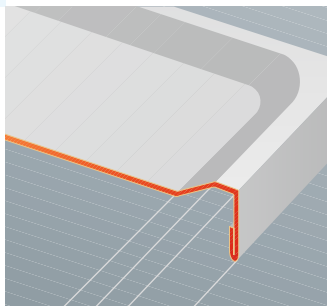
Este gráfico clarifica la forma del pliegue higiénico, con el que están provistos los estantes de todos los carros de servicio HUPFER®. El pliegue higiénico procura no sólo la máxima facilidad de limpieza, sino que protege de heridas durante el proceso de limpieza.
