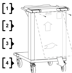
Abb. 6: Rückwand entfernen
